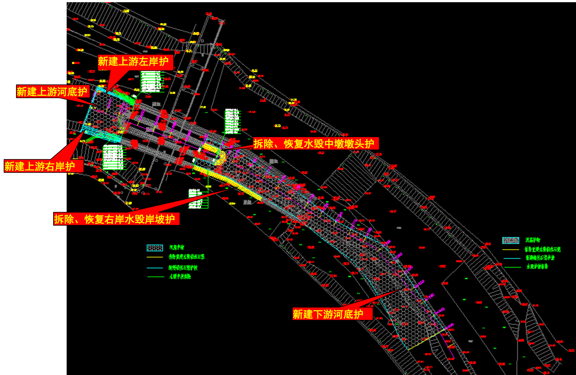
图 1-2 史家口桥下护砌平面布置图
