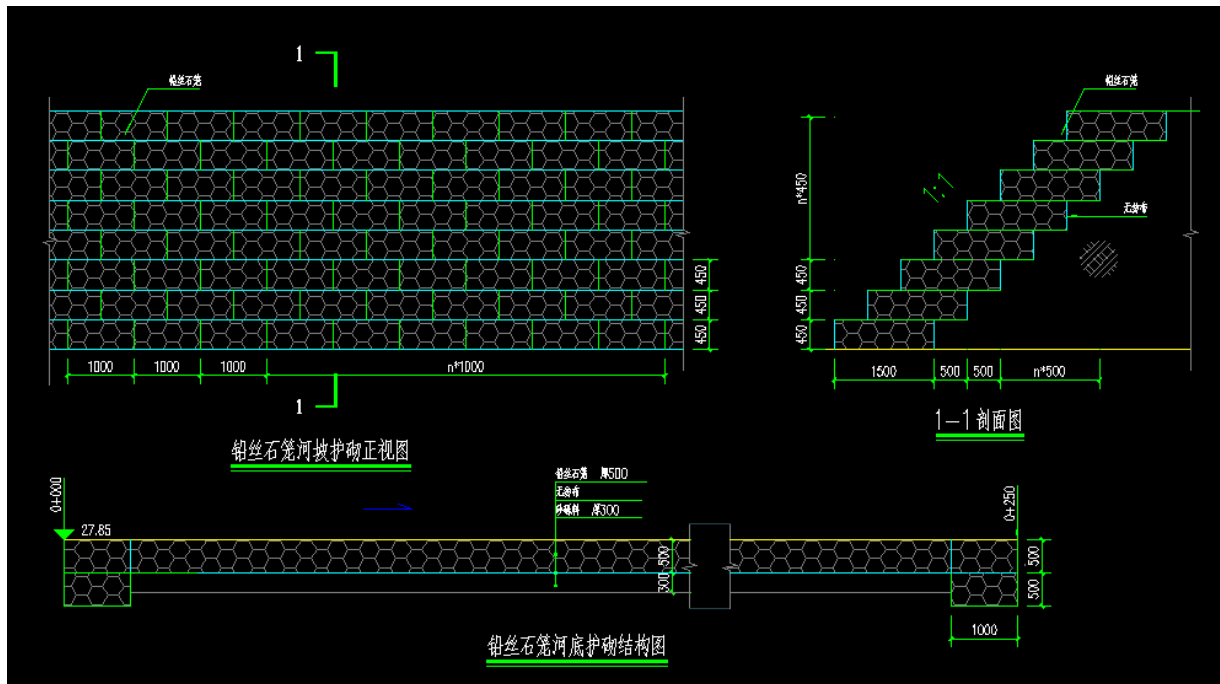
图 4-1 河底、河坡护砌结构图
