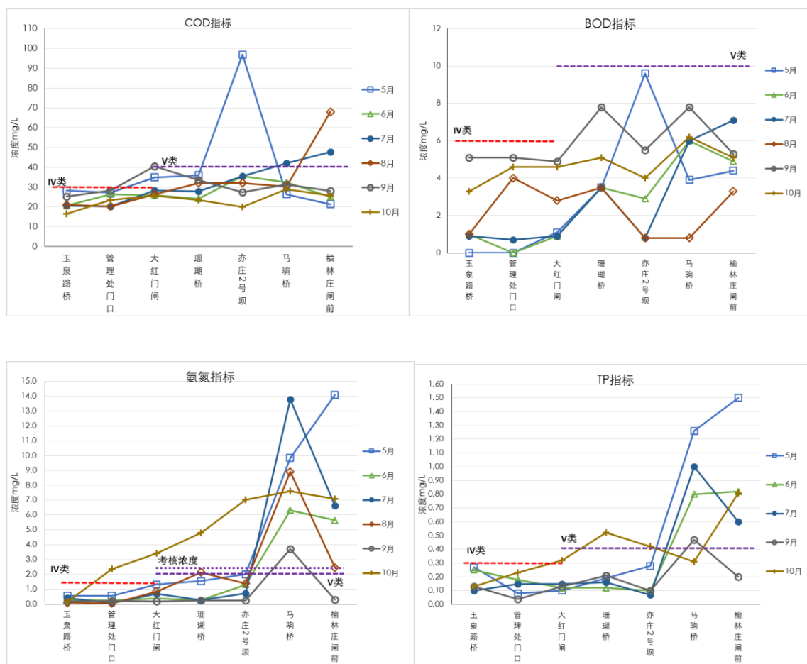
图 1 凉水河不同月份水质沿程变化
