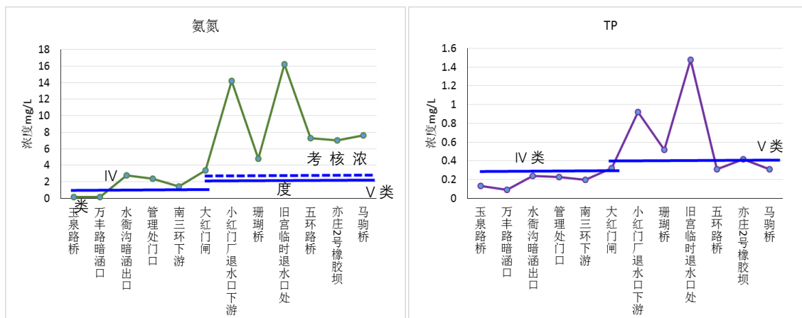
图 2 凉水河 2017 年 10 月水质沿程变化
