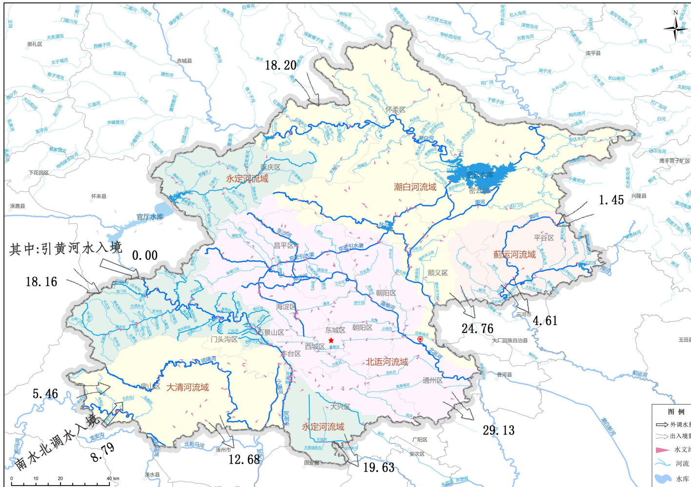
图 2-6 2025 年各水系出、入境水量及调入水量示意图 (单位: 亿 m 3 )
