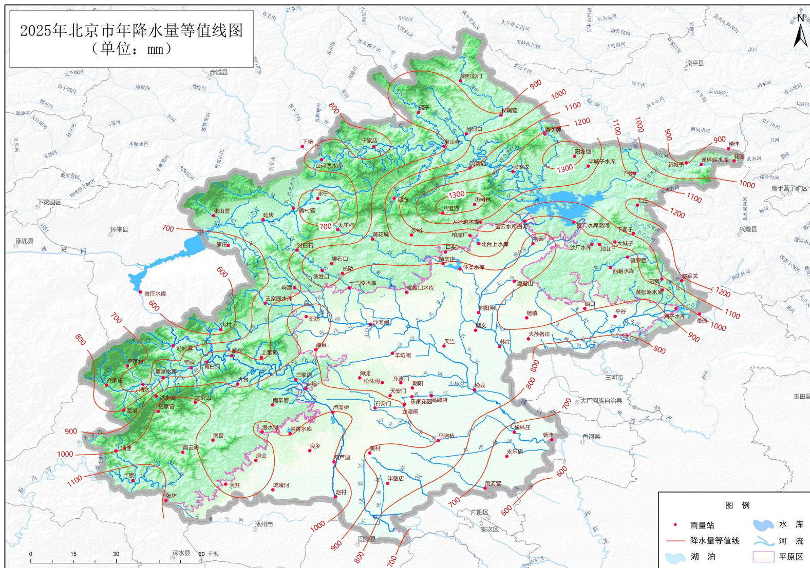
图 2-4 2025 年北京市年降水量等值线图
