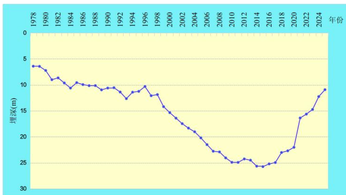
图 2-8 1978-2025 年北京市平原区地下水埋深过程线图
