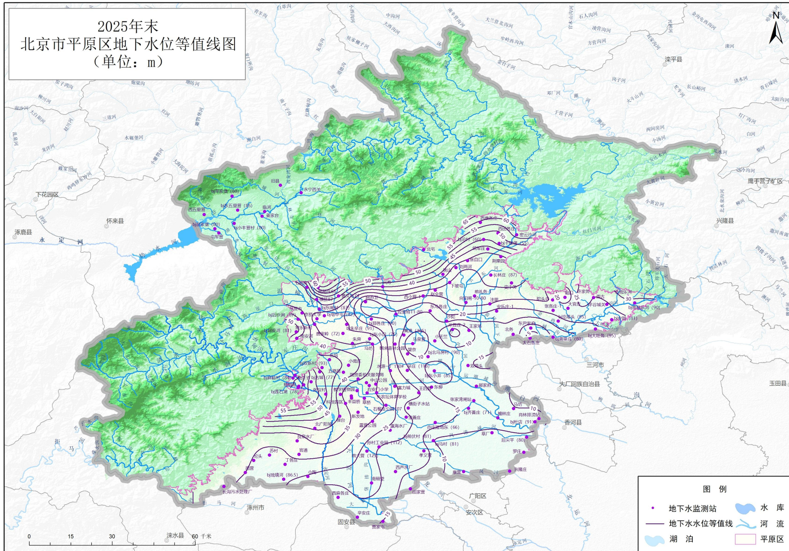
图 2-10 2025 年末北京市平原区地下水水位等值线图
