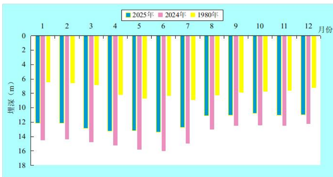
图 2-7 2025 年与 2024 年及 1980 年全市平原区地下水逐月埋深比较图
